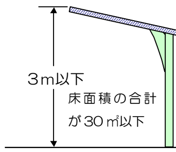
《図② 車庫》
