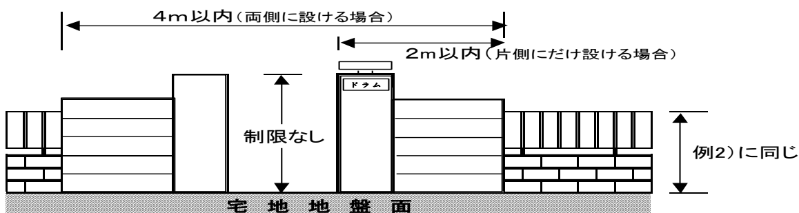
例3) かき又はさくの適用除外される門の例
