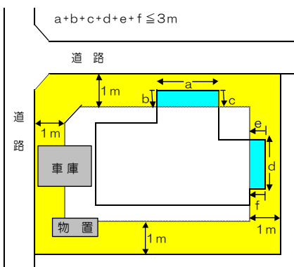
《図①》 外壁又はこれに代わる柱
