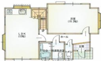
1階 平面図 S:1/100
