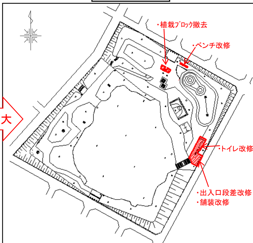
工事箇所図
