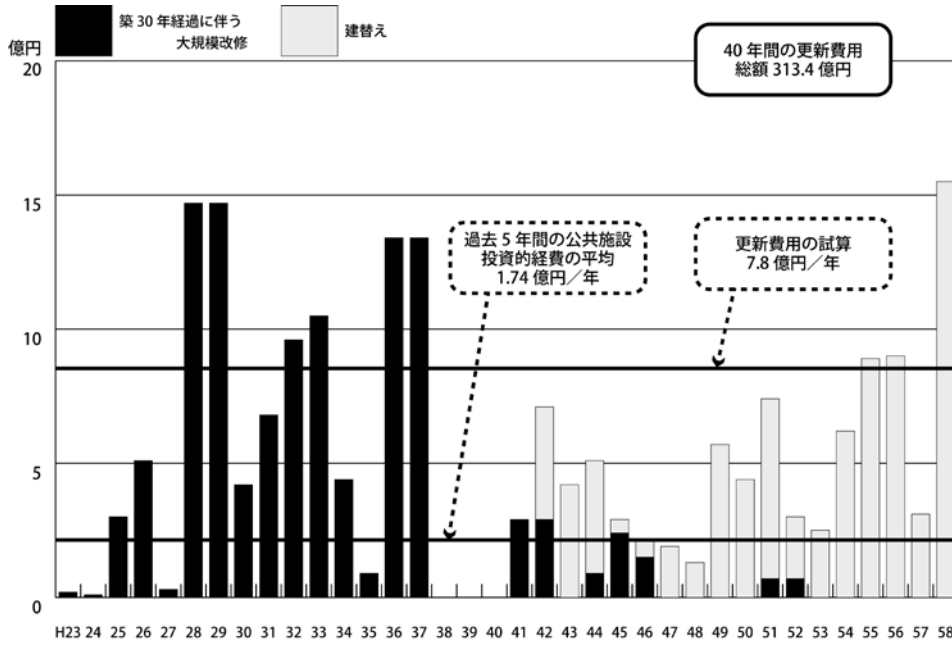
■ 図 1 / 将来更新費用の推計 (公共建築物) 60 年建替えケース
