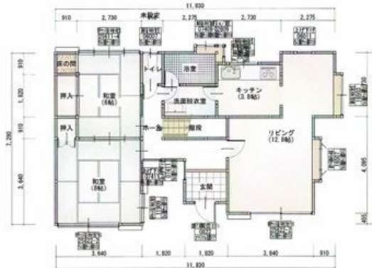
一階平面図
